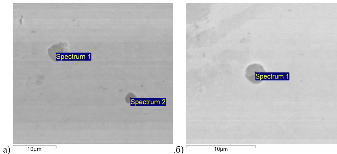
Рис. 12. Химический состав включений образца 13Г1С-У
