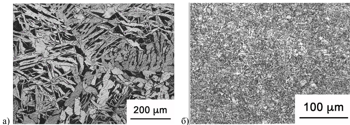
Рис. 6. Структура образцов стали 20КТ, отобранных от НЛЗ и от готовой трубы: а) литая видманштеттова; б) бейнит.
