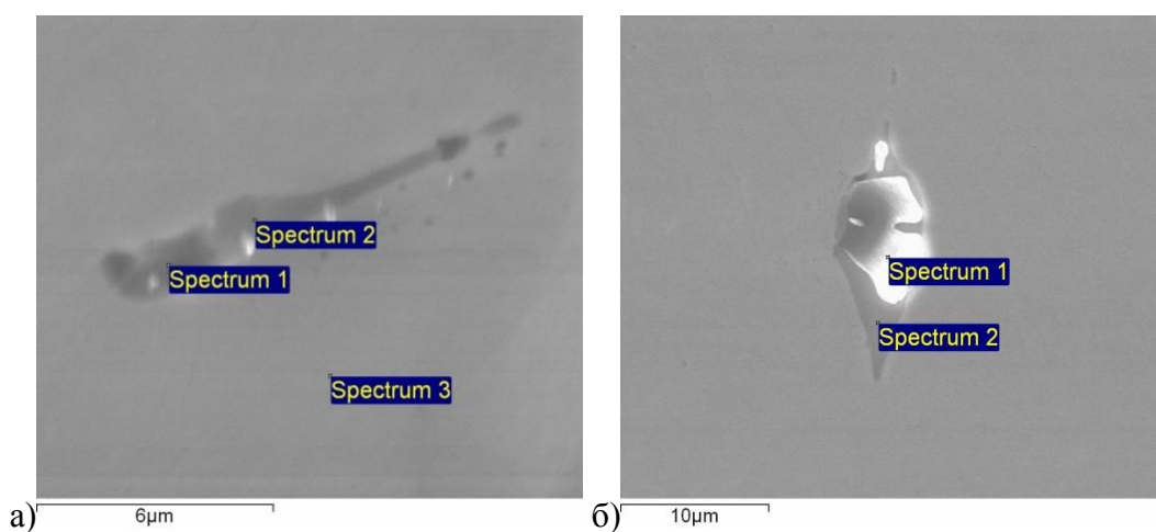
Рис. 9. Неметаллические включения образца 17ГС.
